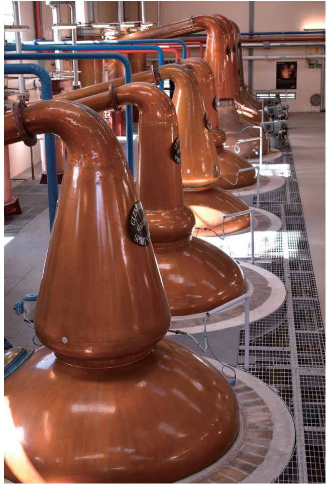
第2蒸留棟のポットスチル。 初留は今もガス直火だ。
